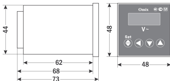
Рис. 3 – Размеры. Тип корпуса P44
